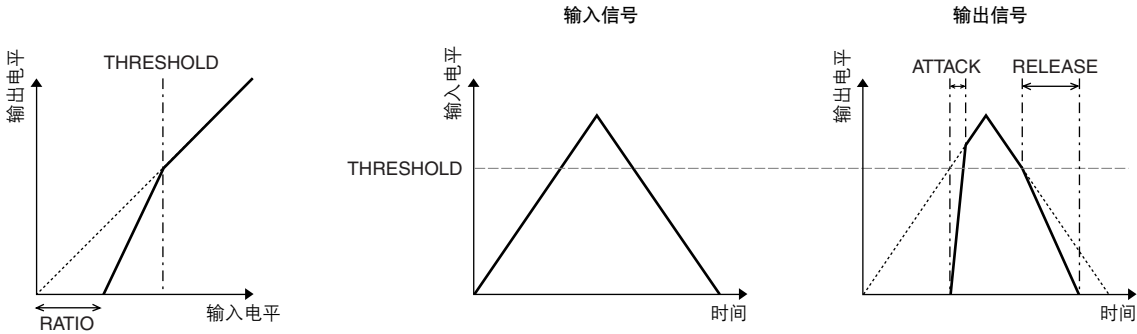
I/O 特征 (KNEE= 硬, OUT GAIN=0.0dB)
